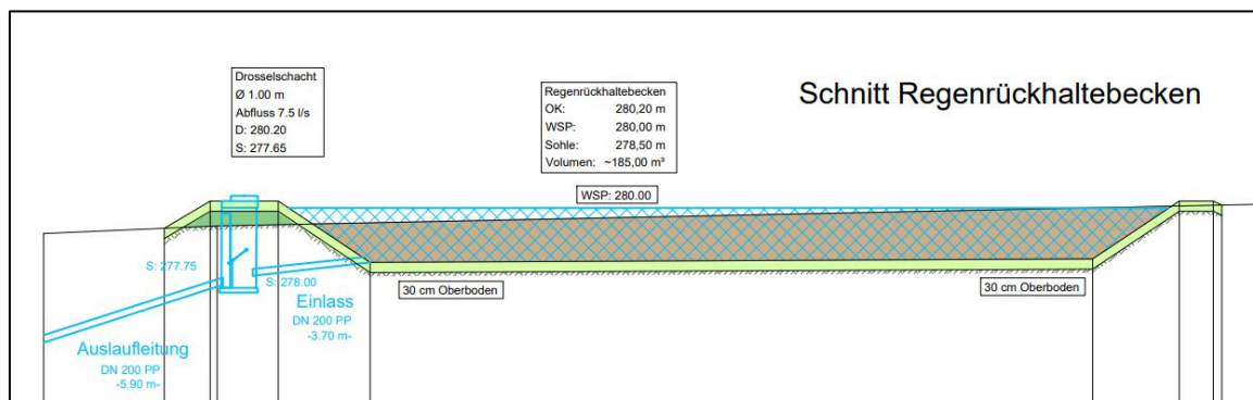
Abbildung 2: Auszug Entwässerungsplanung 2024
